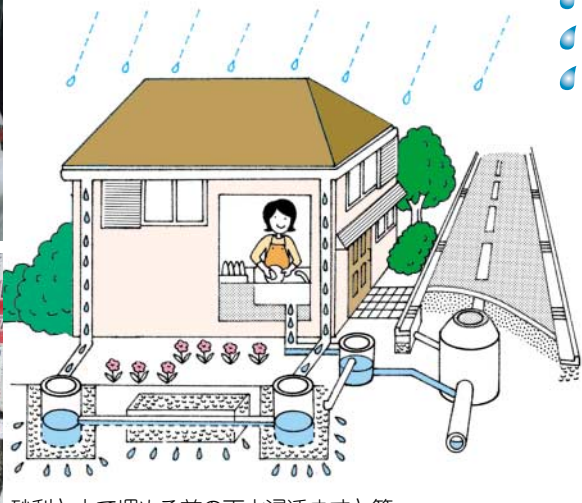
砂利と土で埋める前の雨水浸透ますと管。雨水がますや管の穴から地中へ浸透していきます。
