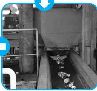
投入されびんはコンベアに送られ…
