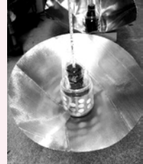
簡易ソーラークッカー
