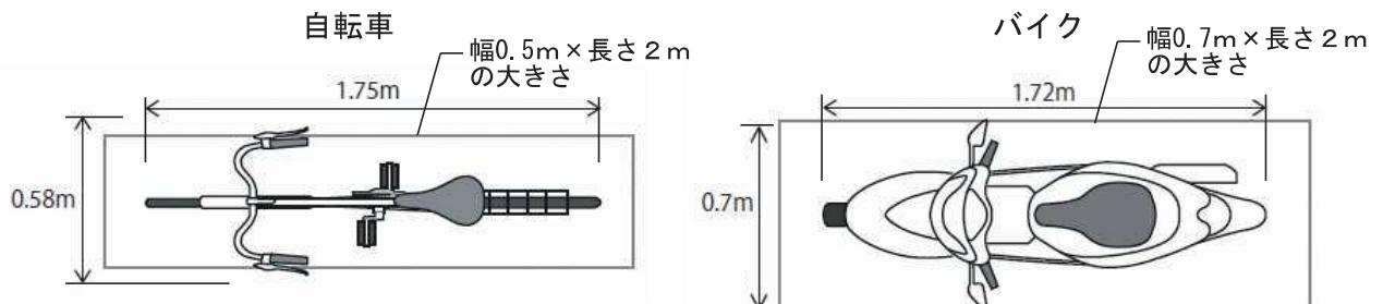
参考図10-2 一般的な自転車およびバイク（原動機付自転車）の寸法の目安
