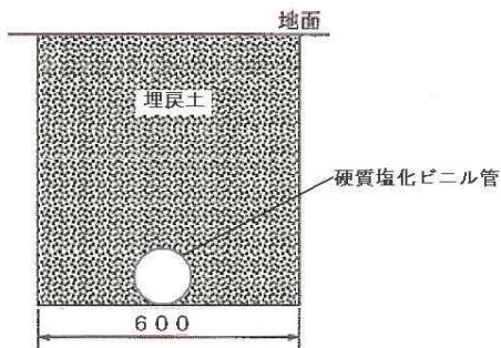
接続管
