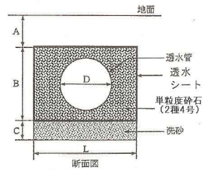
浸透地下埋設管
