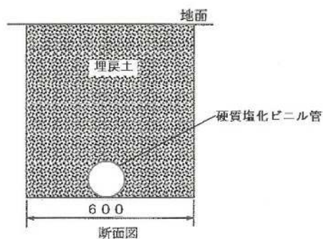
接続管
