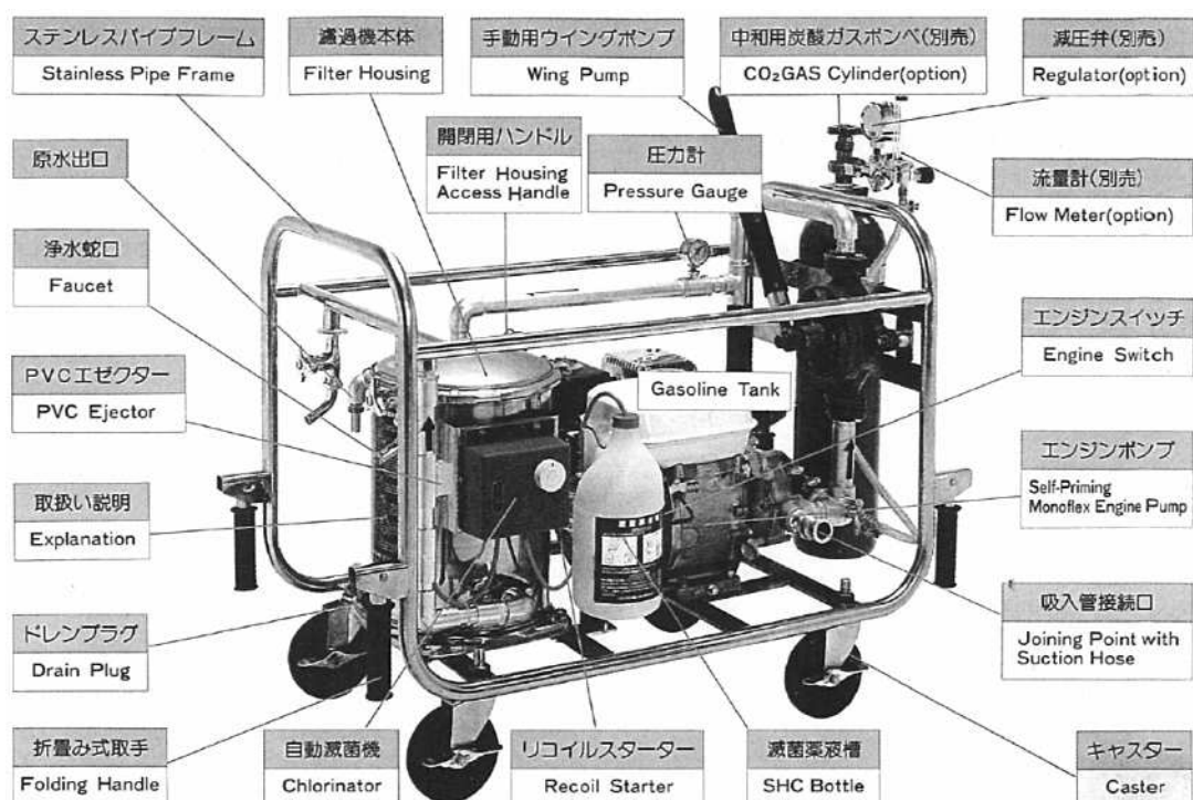
自動式ろ過機各部名称
