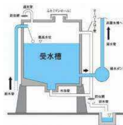
受水槽の構造（模式図）
