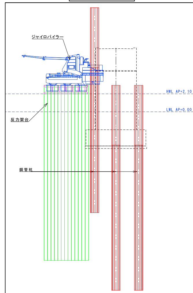
断面図
