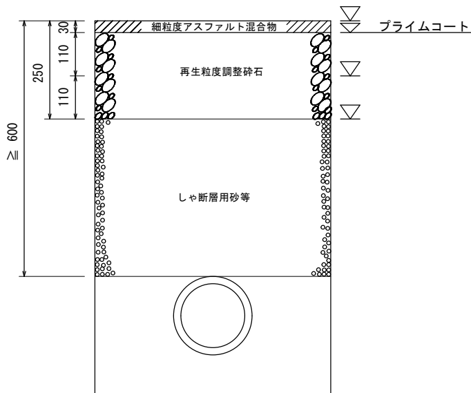
(1) アスファルトコンクリート舗装 25型
