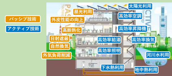
パッシブ技術とアクティブ技術を組み合わせたZEBのイメージ (出典：環境省HP)
