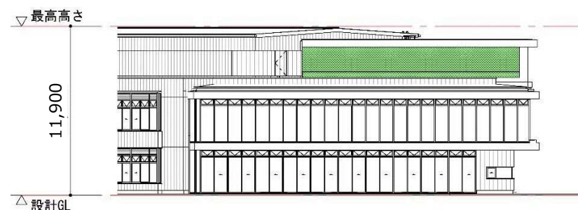
西側立面図
