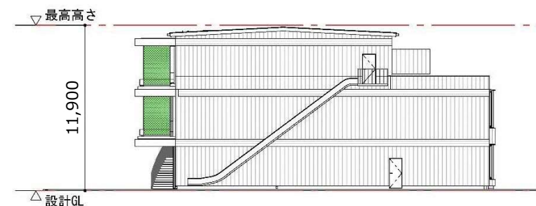
東側立面図
