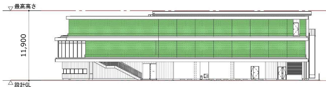
南側立面図
