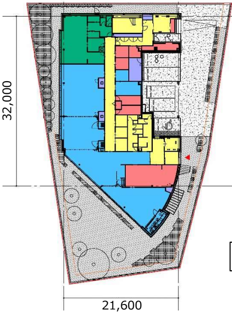
3 階平面図
