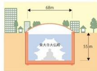
LNGタンクの内部の図
