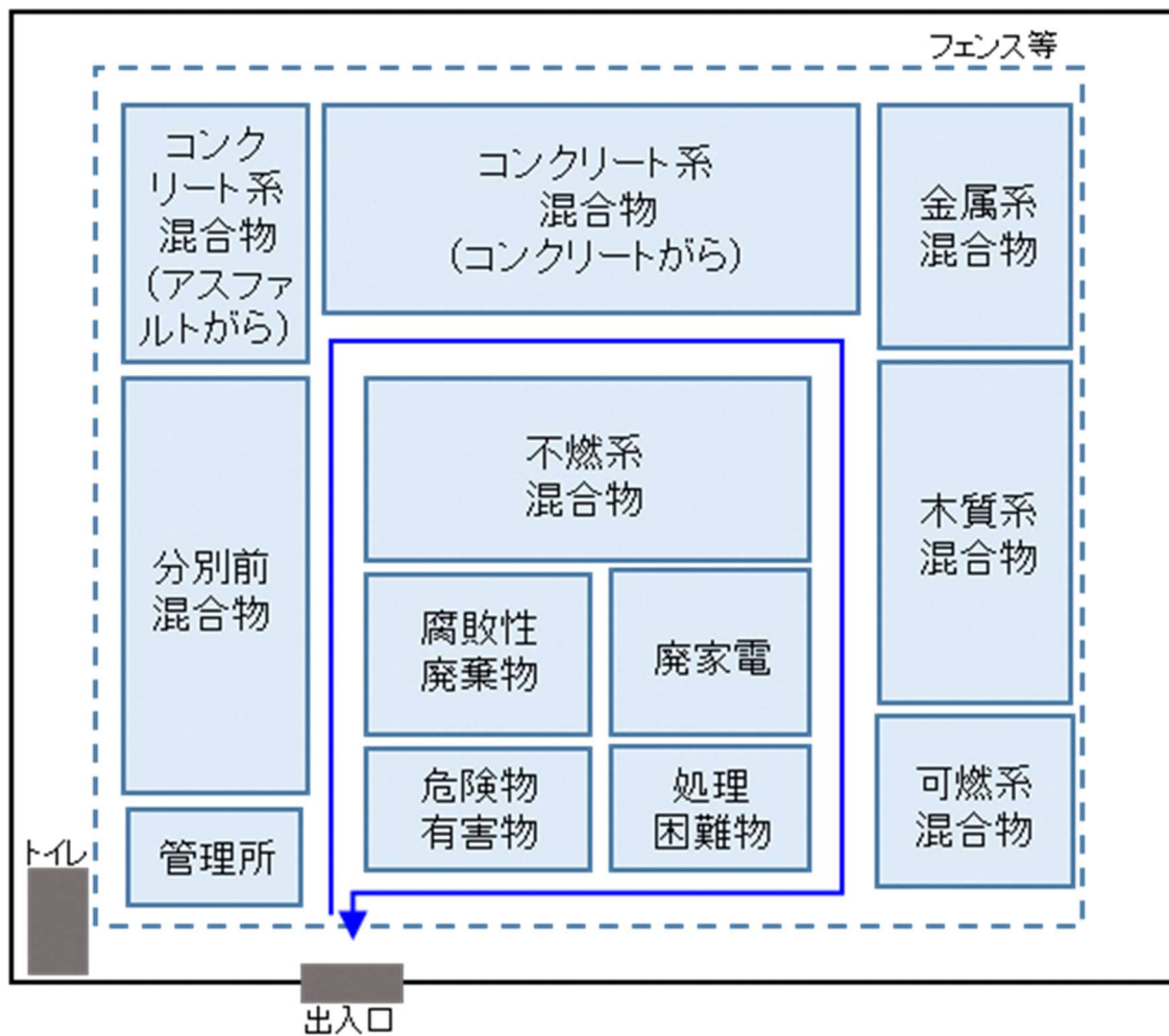
図 一次仮置場レイアウト例 【資料編：資料5. 仮置場等のレイアウト（例） 2. 一次仮置場のレイアウト（例）】
