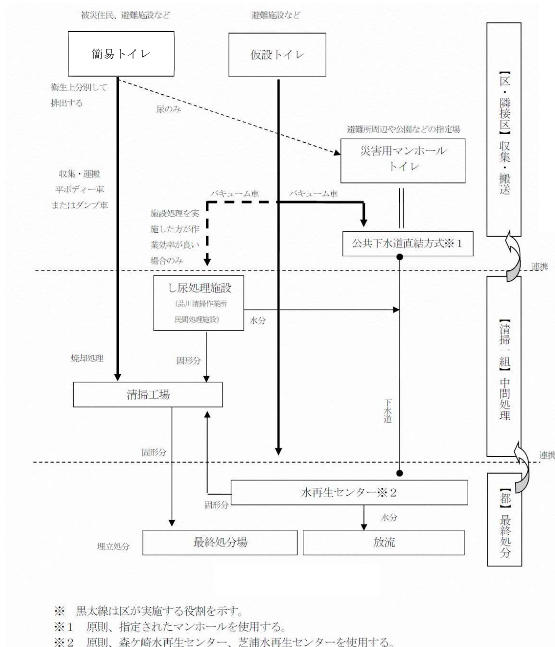
図表3-38 し尿処理に係る対応の流れ
