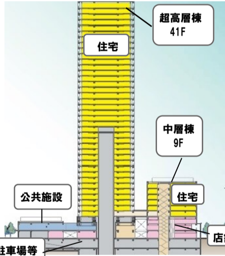
【建築物断面イメージ】 (出典:武蔵小山駅前通り地区市街地再開発組合)
