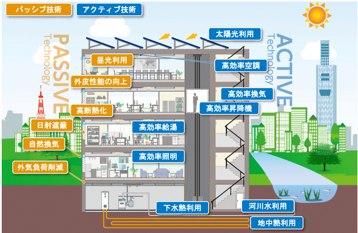
図表 2-27 パッシブ技術とアクティブ技術を組み合わせたZEBのイメージ (出典：環境省 HP)
