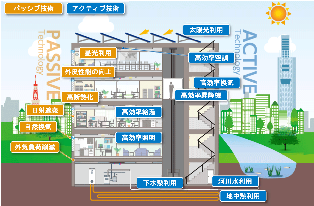
図表 2-27 パッシブ技術とアクティブ技術を組み合わせた Z E B のイメージ (出典：環境省 HP)
