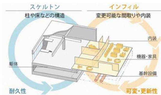
図表 2-28 スケルトン・インフィル工法イメージ（出典：中野区 HP）
