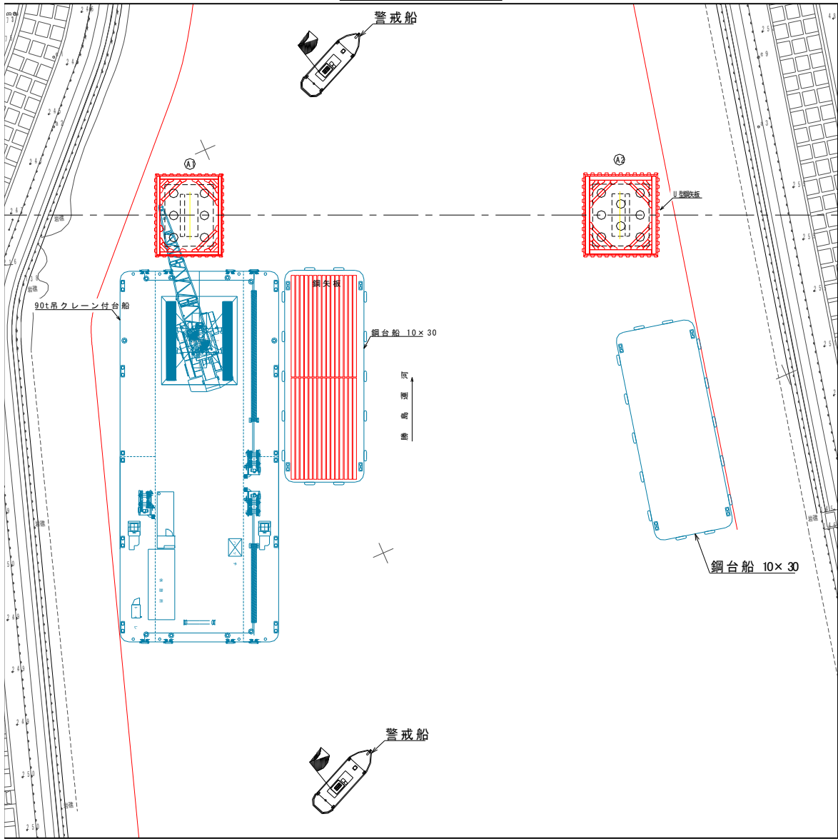
平面图
