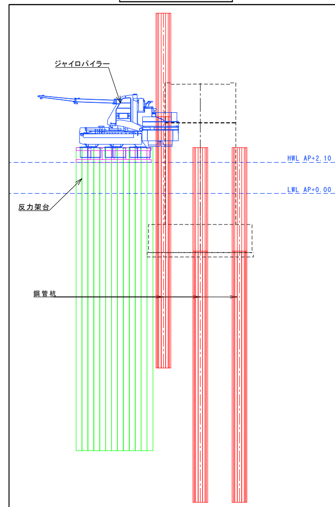
断面図
