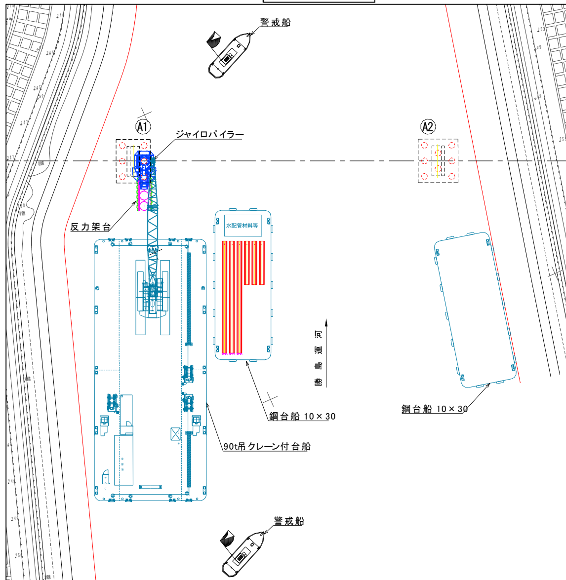
平面図
