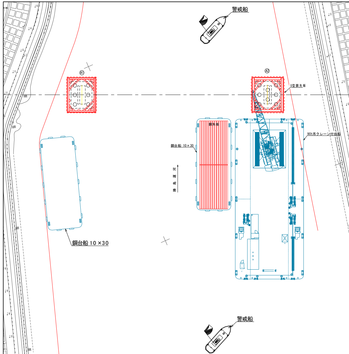
平面図
