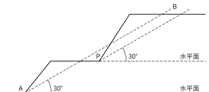
図 0-6 別の崖とみなすケース
