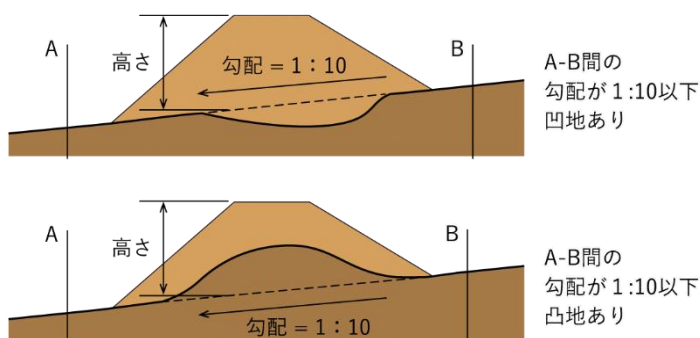
図 0-26 堆積地盤の一部に凹凸がある場合の堆積高さの考え方
