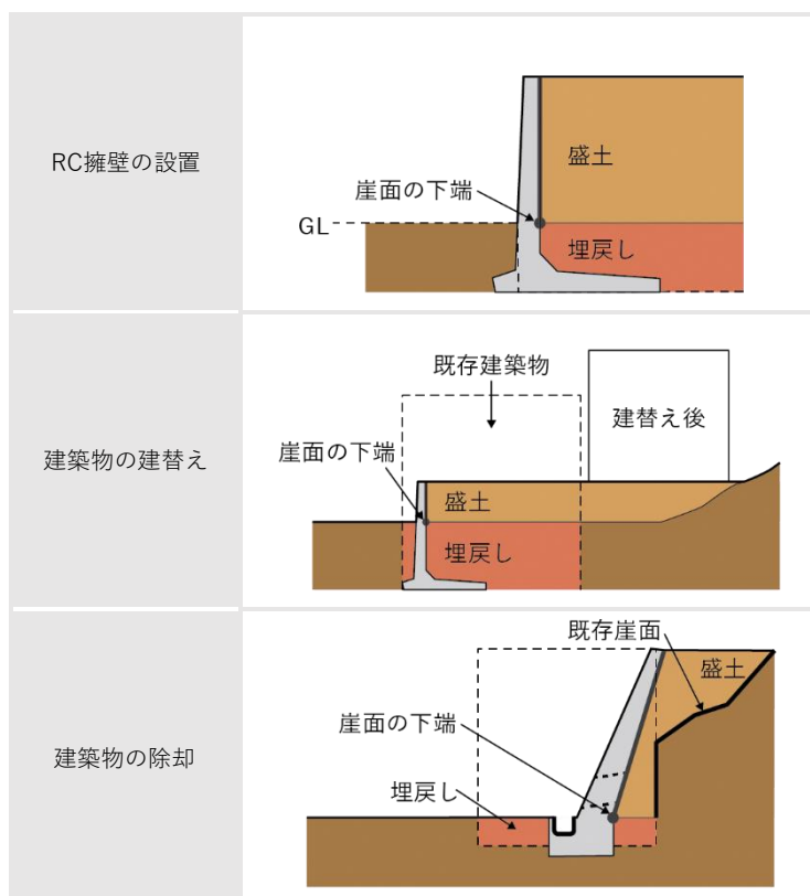
図 0-4 盛土と埋戻し
