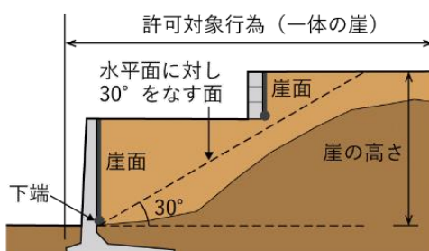
図 0-12 崖の高さ（一体の崖）
