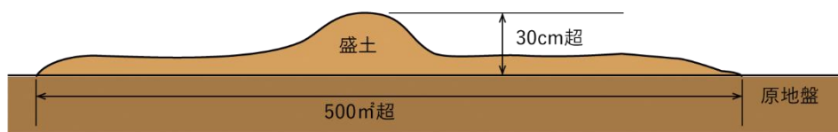
図 0-19 盛土または切土する土地の面積が 500m 2 超で、盛土または切土をする前後の地盤面の標高の差が 30cm 超となる場合イメージ
