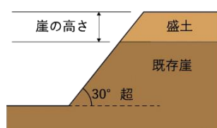
図 0-10 崖の高さ（盛土）
