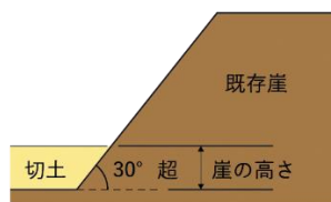
図 0-11 崖の高さ（切土）
