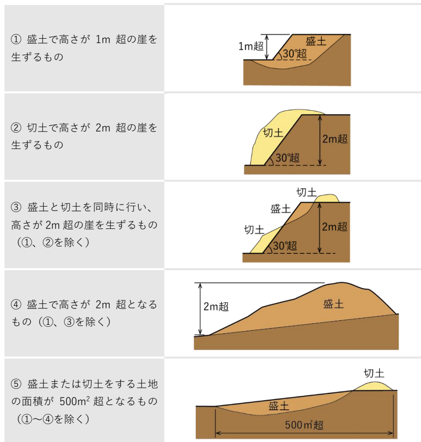
図 0-3 土地の形質変更（盛土・切土）の定義
