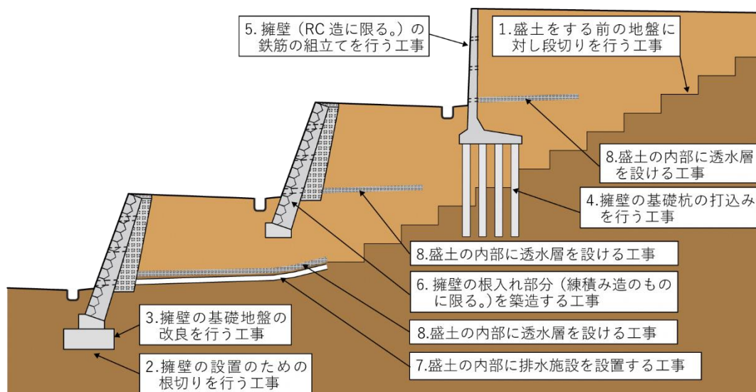
図 0-1 中間検査の対象となる工事のイメージ
