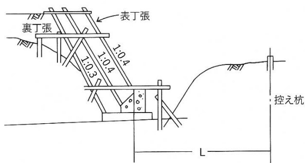
図 0-4 丁張りの設置例
