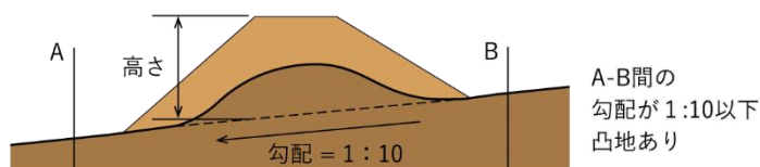
図 0-6 原地盤に極端な凹凸がある場合
