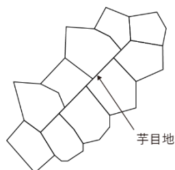
図 0-5 芋目地の組積みの例（施工してはならない積み方）
