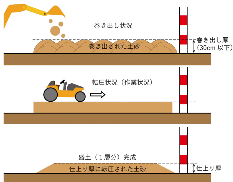
図 0-2 巻き出しと転圧の方法
