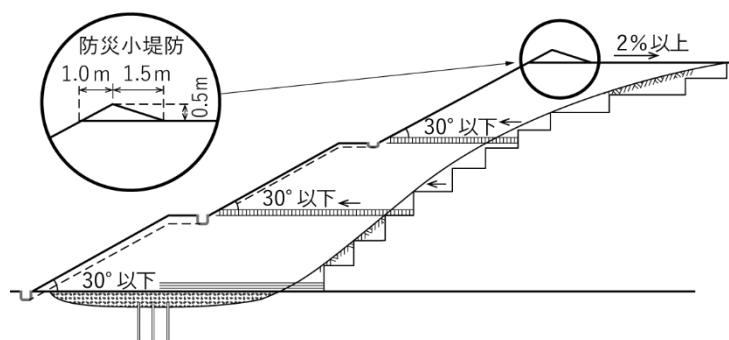
図 0-3 防災小堤
