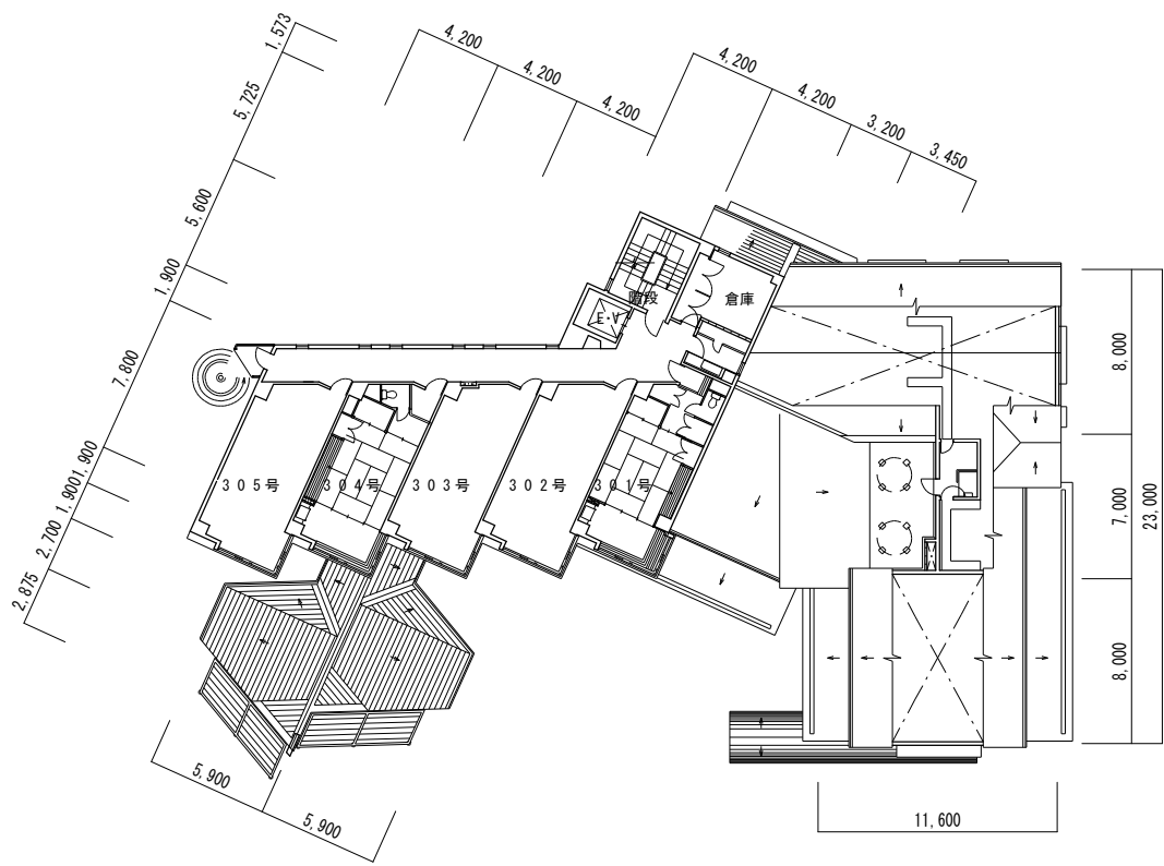
3階平面図 S = 1 : 4 0 0
