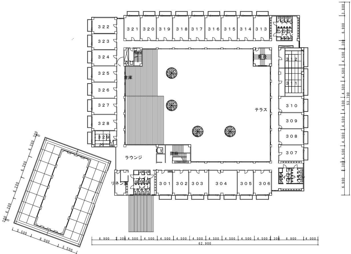
3階平面図 S = 1 : 6 0 0
