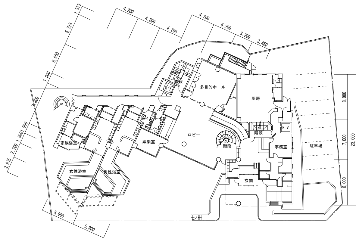
1階平面図・配置図 S = 1 : 4 0 0
