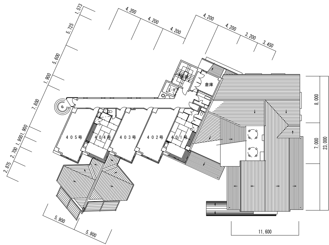
4階平面図 S = 1 : 4 0 0
