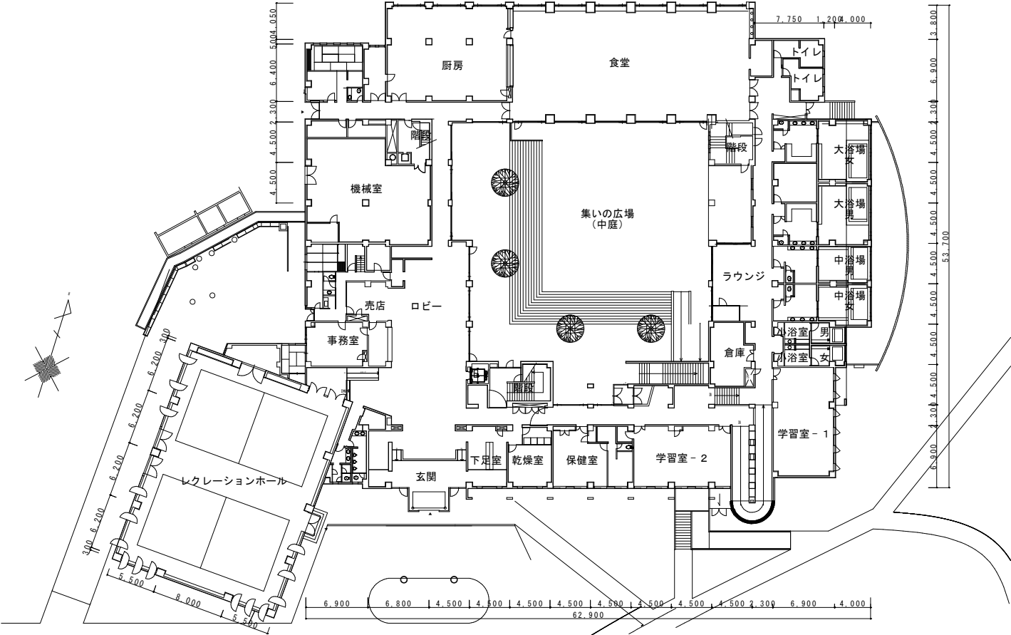
1階平面図 S = 1 : 6 0 0
