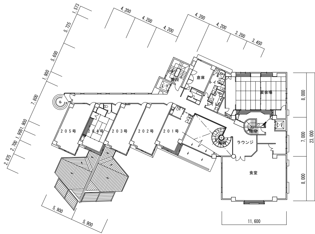
2階平面図 S = 1 : 4 0 0
