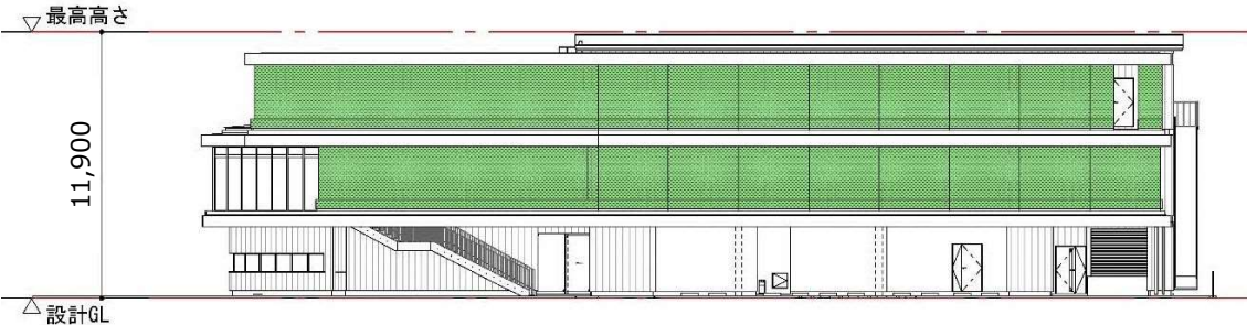
南側立面図
