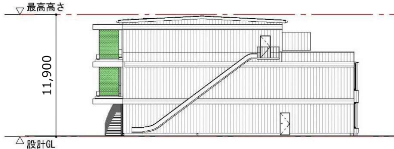
東側立面図
