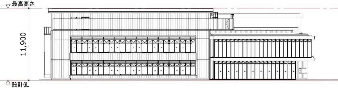
北側立面図
