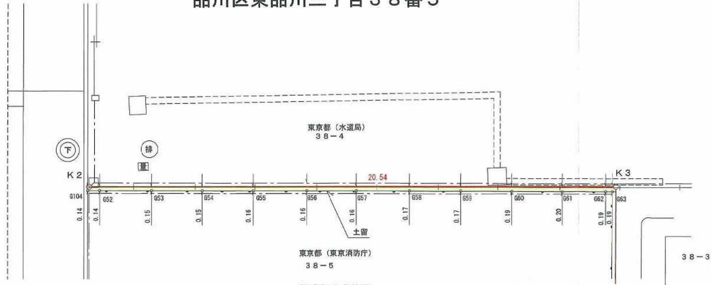
越境部分求積図
