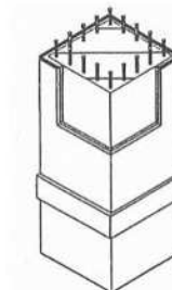
鋼板巻きによる柱の補強イメージ
