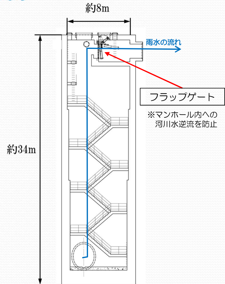
人孔（マンホール）断面図
