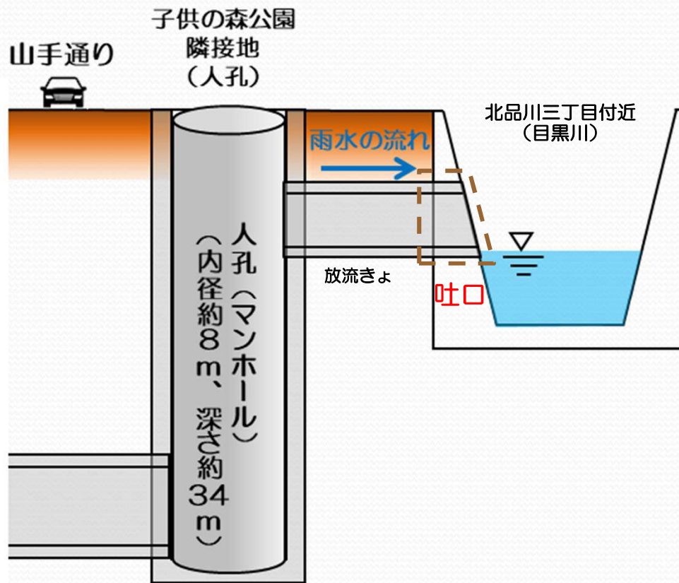
吐口の位置関係
