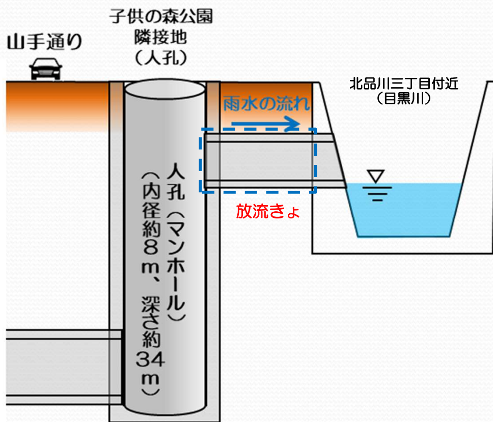
放流きよの位置関係
