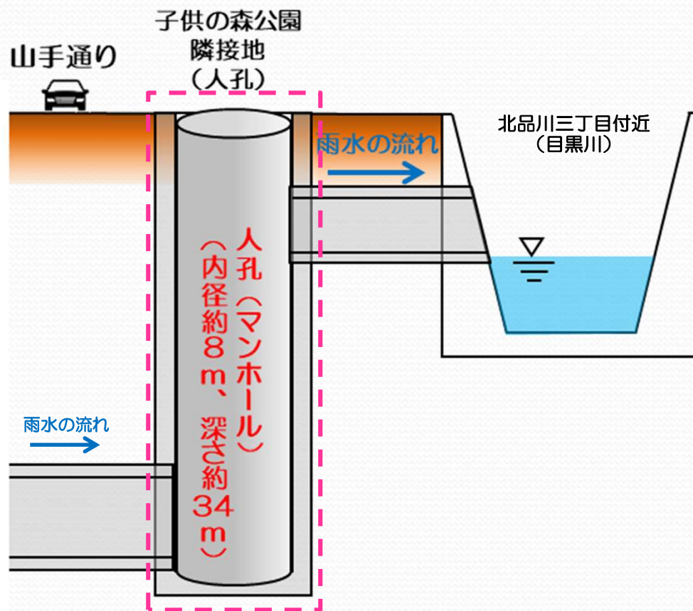
人孔（マンホール）の位置関係
