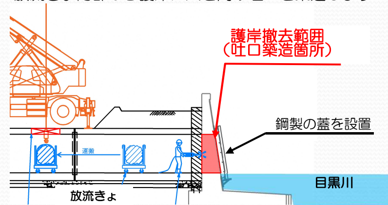
護岸穴開け作業イメージ図
