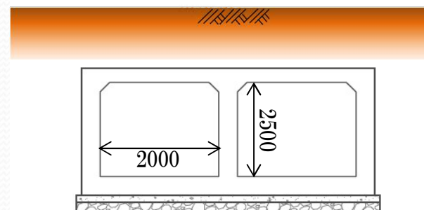
放流きよA-A断面図
