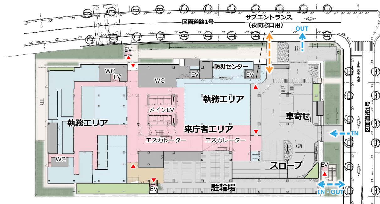
1階
