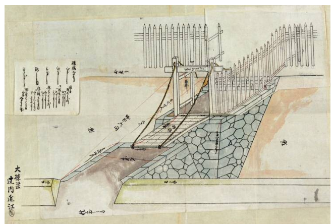
▲御殿山英国公使馆可收放的桥梁（《品川五外国公使馆工程图面》收录图，东京都立中央图书馆东京志料文库藏品）
