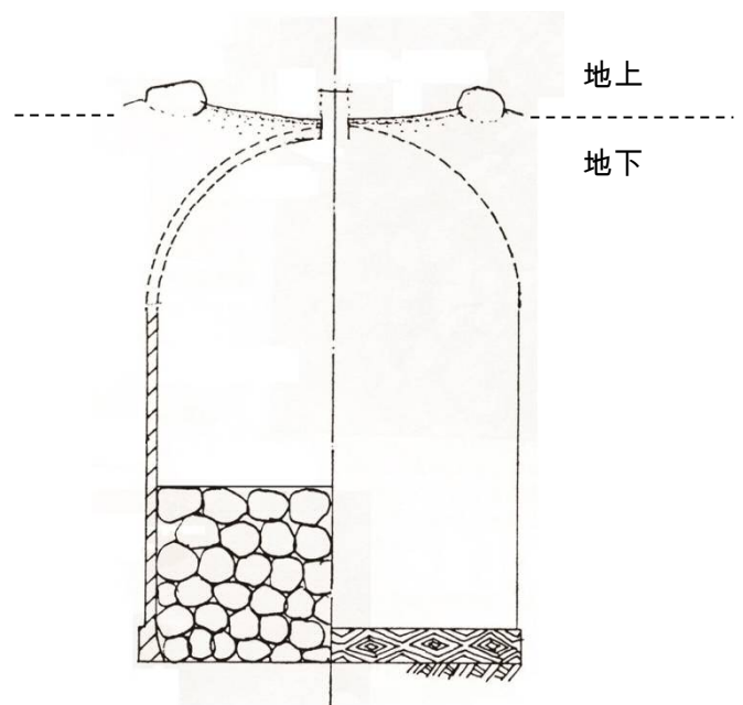
▼水琴窟的剖面圖
