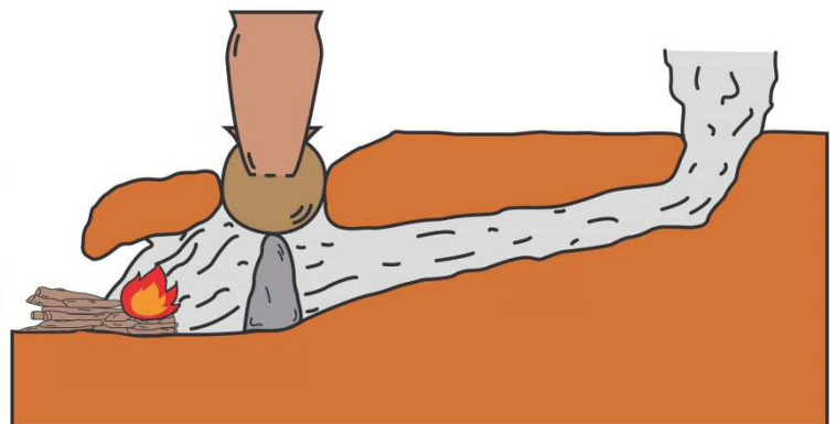
▲爐灶斷面圖
